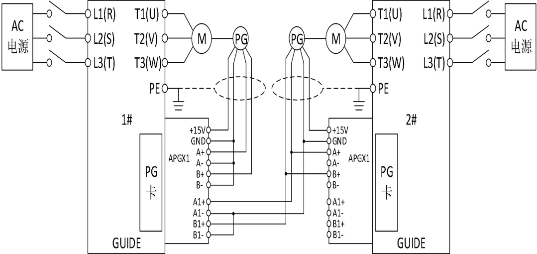
编码器为单端输出信号的接线示意图
