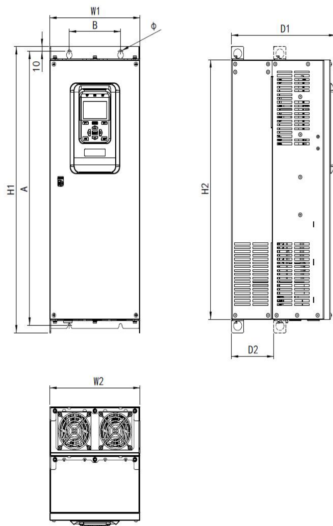
N4 机型尺寸及安装尺寸示意图
