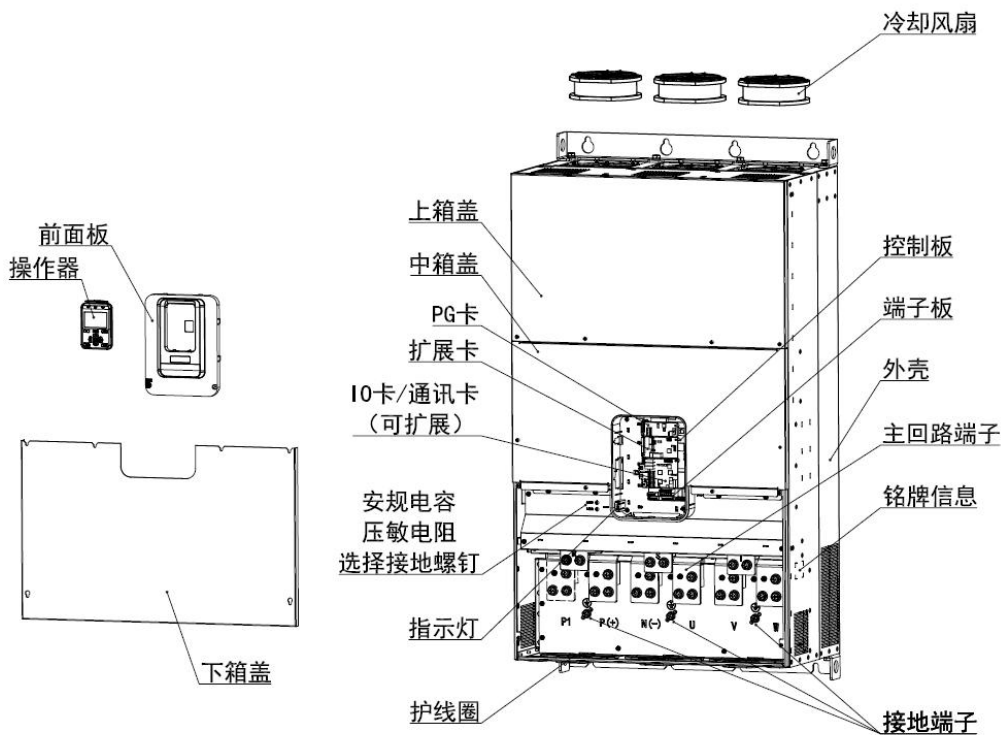
N10 产品部件示意图 (三相 380V~480V, 315kW~400kW)
