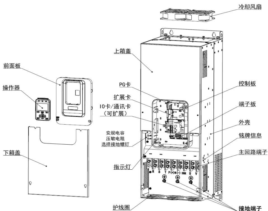
N6 产品部件示意图 (三相 380V~480V, 90kW~110kW)
