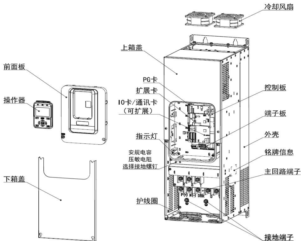
N5 产品部件示意图 (三相 380V~480V, 45kW~75kW)
