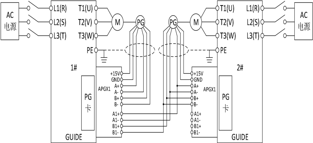
编码器为差分输出信号的接线示意图
