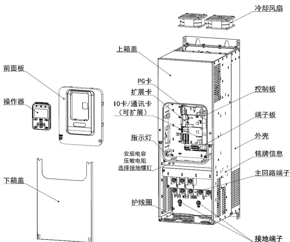
N4 产品部件示意图 (三相 380V~480V, 22kW~37kW)
