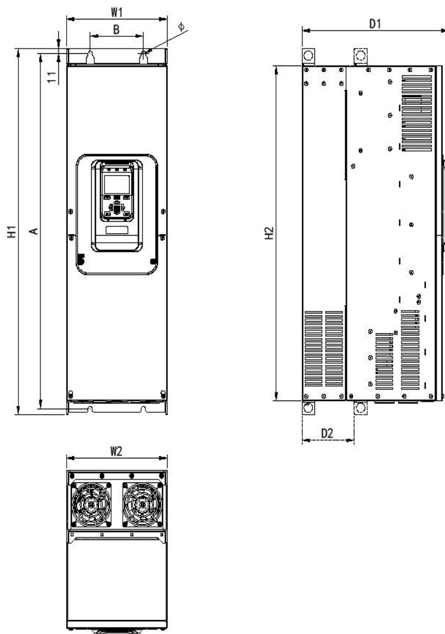
N5~N6 机型尺寸及安装尺寸示意图
