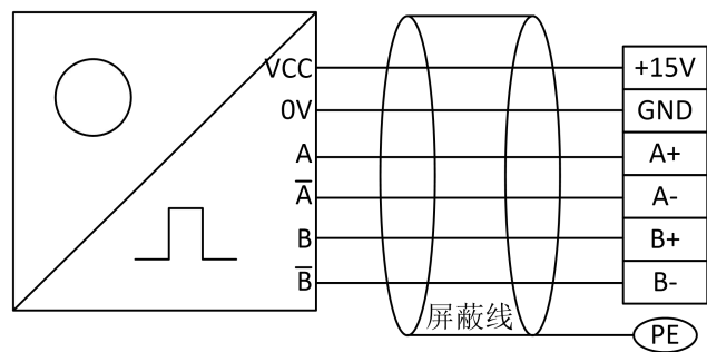
常用推挽输出（差动接线方式）编码器应用举例：
