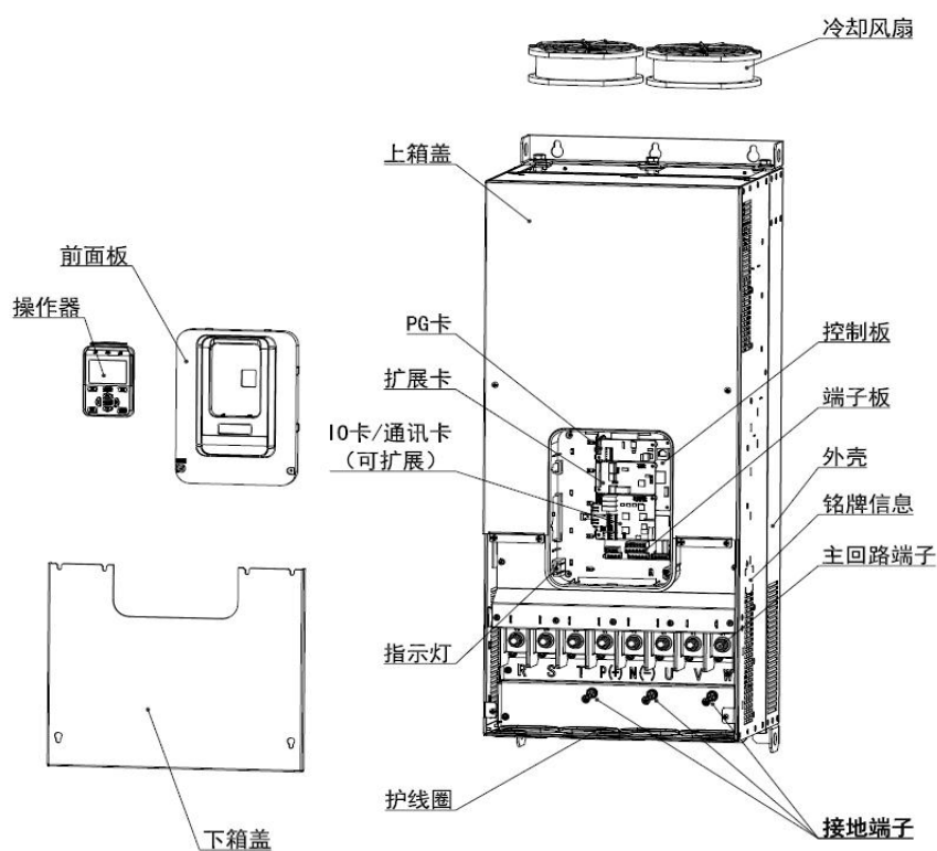
N7 产品部件示意图 (三相 380V~480V, 132kW~160kW)
