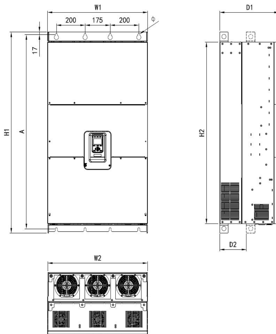
N10 机型尺寸及安装尺寸示意图
