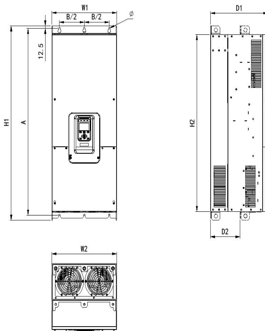
N7~N9 机型尺寸及安装尺寸示意图
