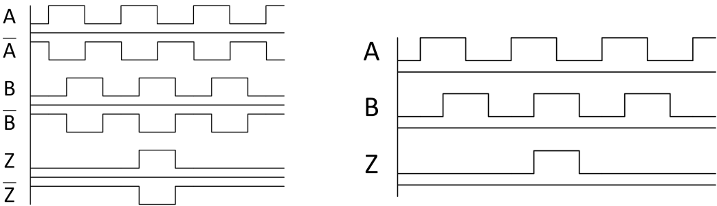
编码器差分输出信号
