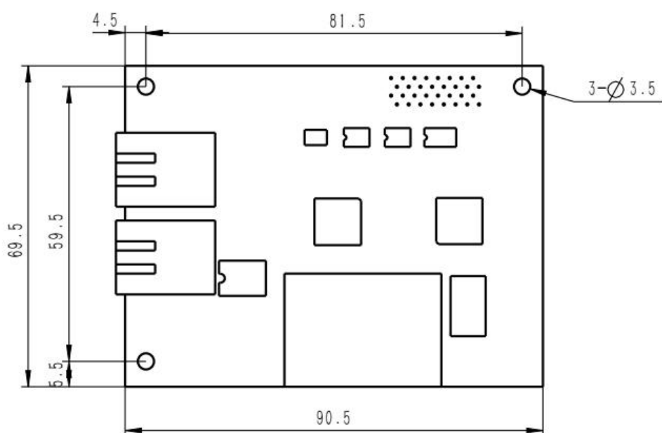
PROFINET 模块尺寸（单位 mm）
