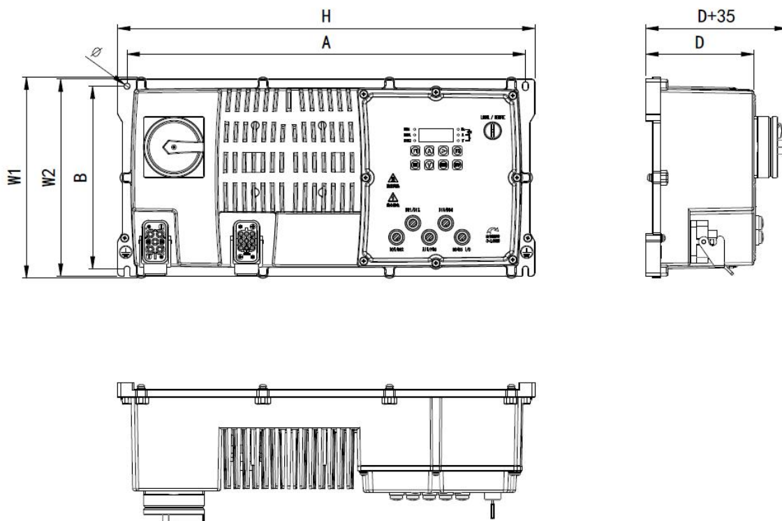
N1 机型：0.7-2.2kW 外型尺寸及安装尺寸示意图（无风扇）
