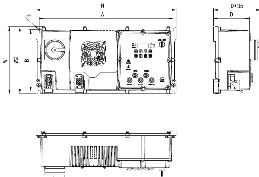
N2 机型：3.7-5.5kW 外型尺寸及安装尺寸示意图（有风扇）
