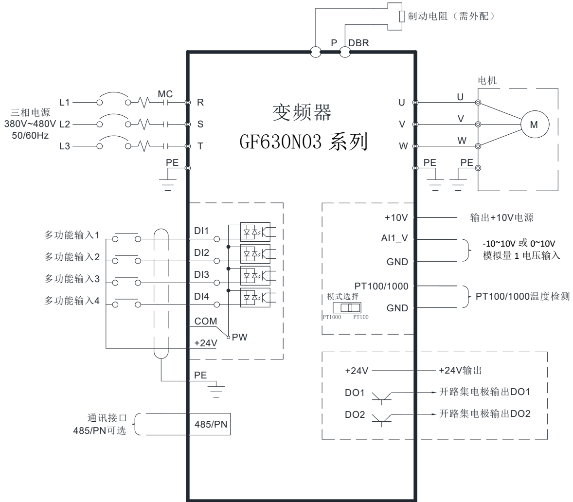
三相 380~480V 典型接线图
