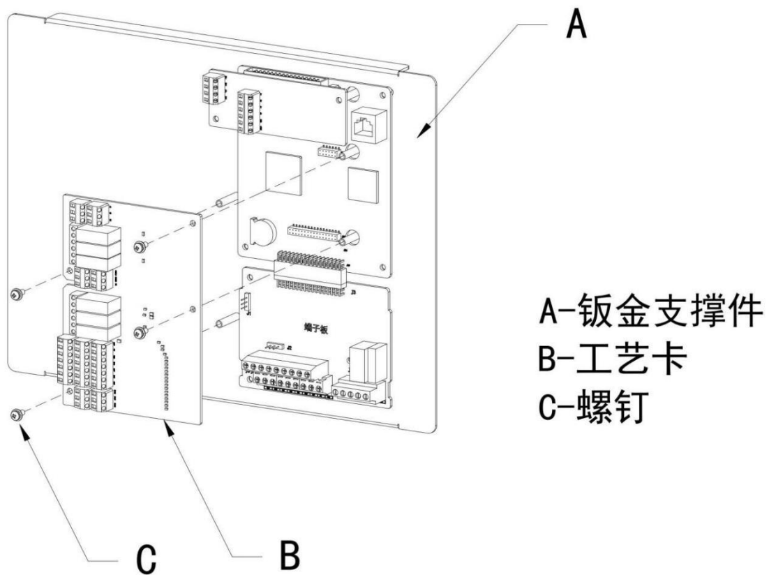
工艺卡的安装
