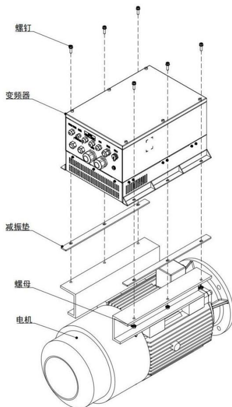
起升变频器安装示意图
