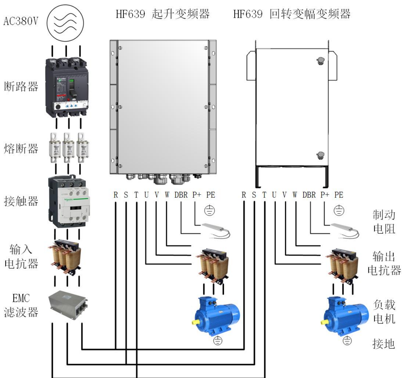
HF639 变频系统外围电气元件的使用说明
