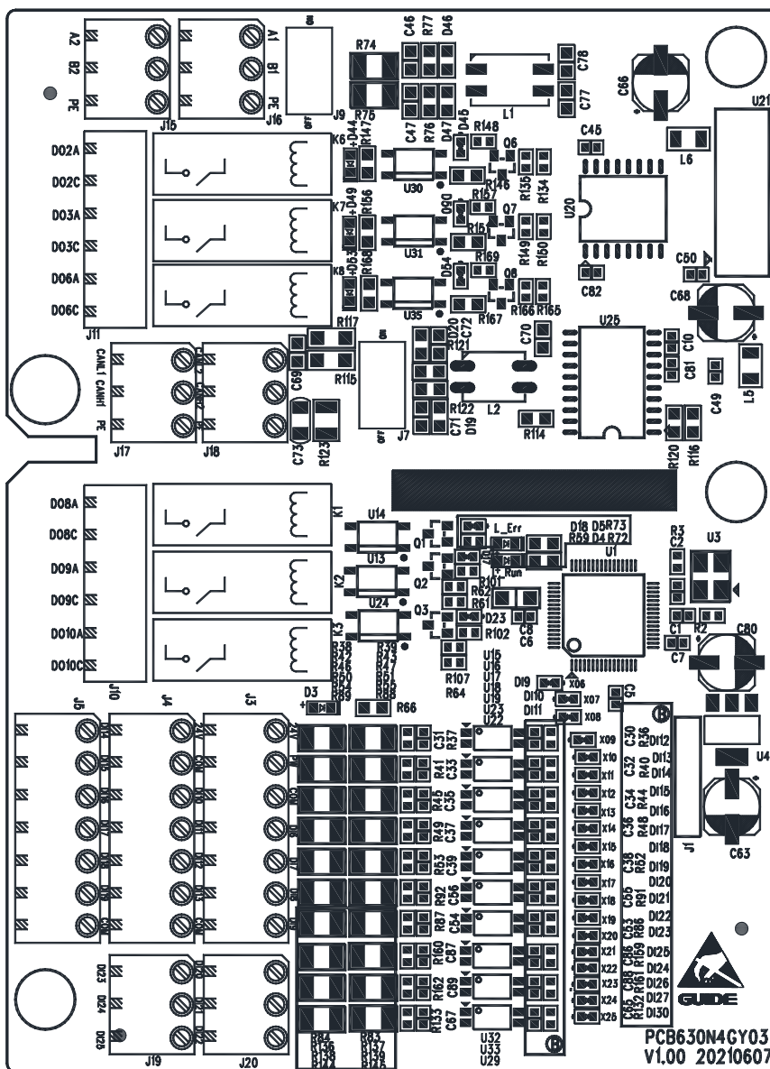
GDHF-AGYZ1 工艺卡布局图
