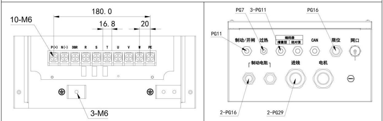
回转变幅变频器端子分布图
