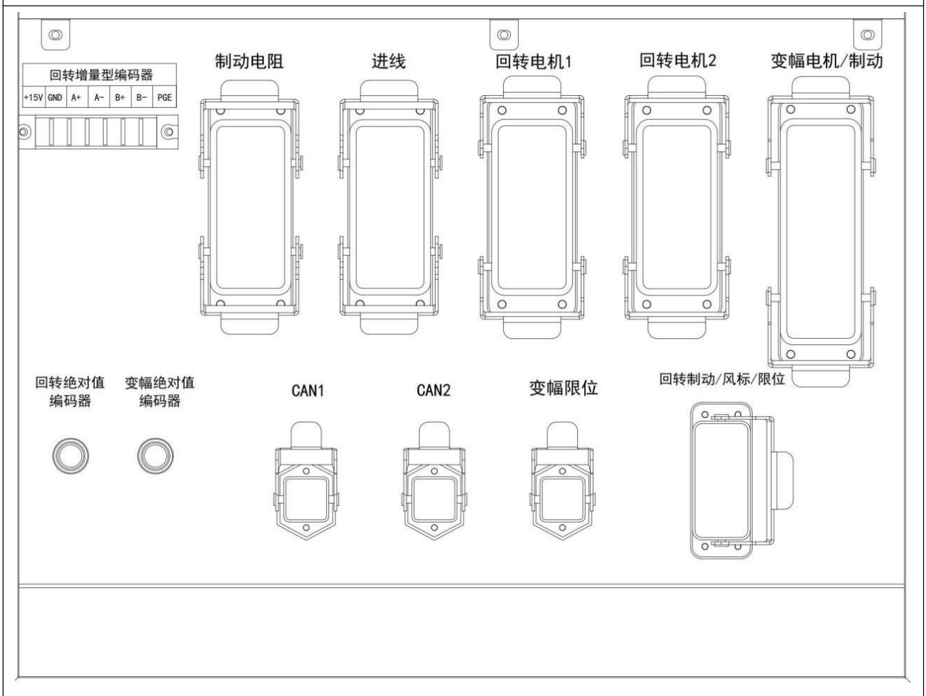
回转变幅变频器端子分布图
