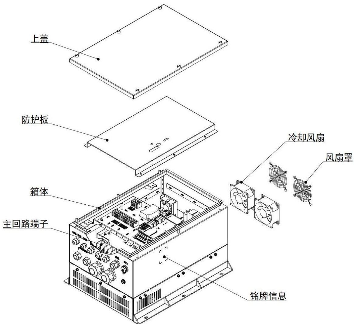
起升变频器部件示意图
