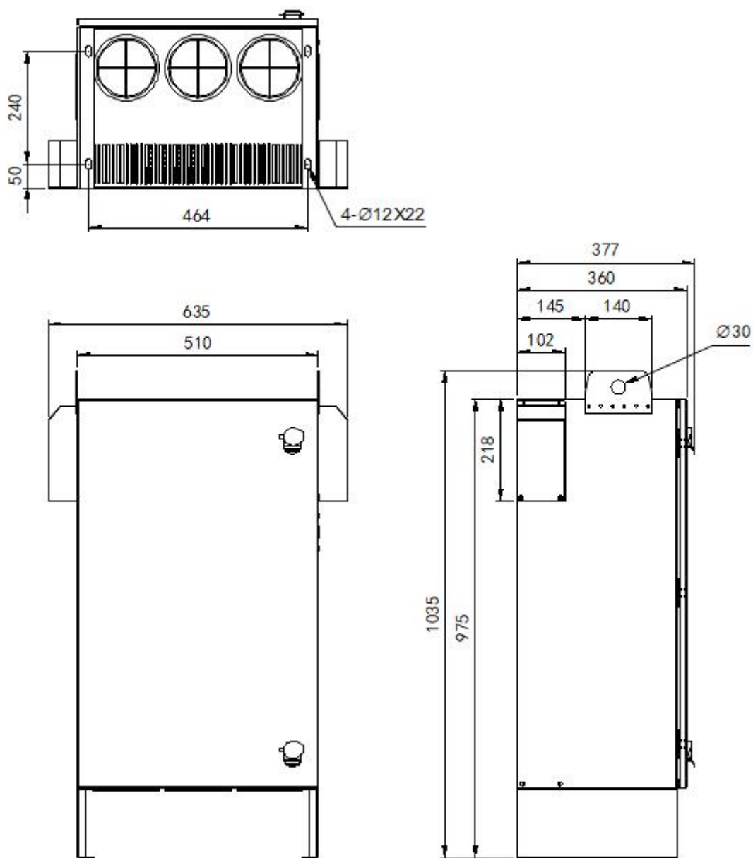
回转变幅变频器尺寸及安装尺寸示意图
