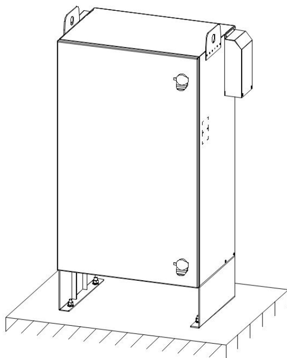
回转变幅变频器安装示意图
