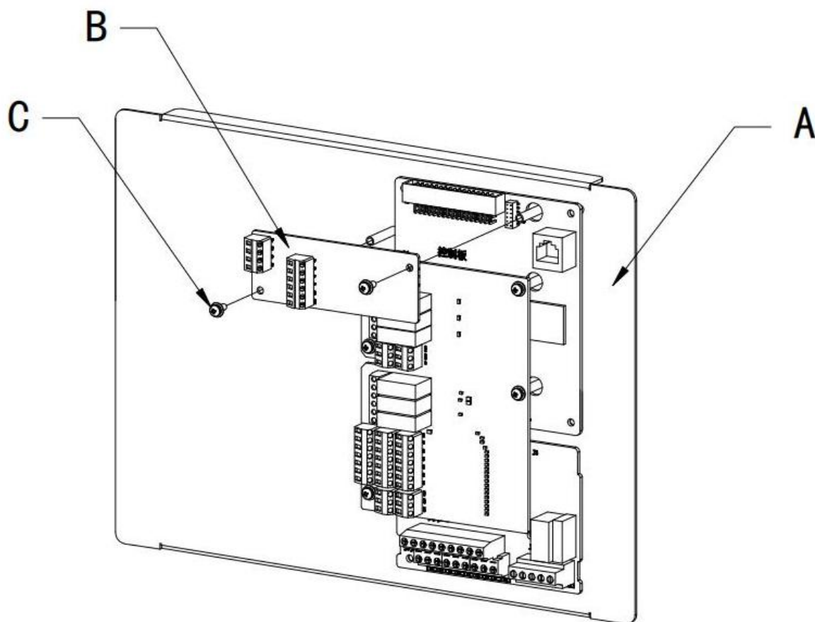
A: 钣金支撑件 B: PG 卡 C: 螺钉
