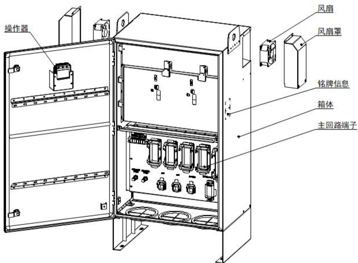
回转变幅变频器部件示意图
