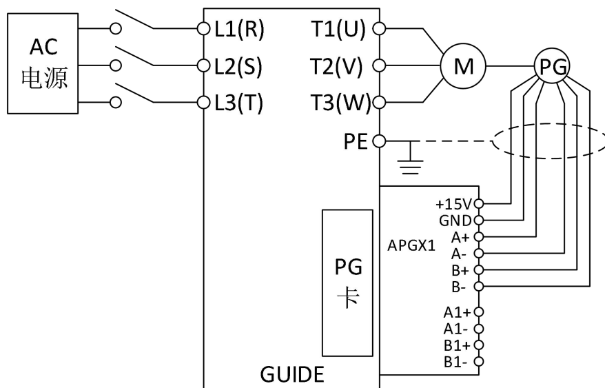
接线原理示意图
