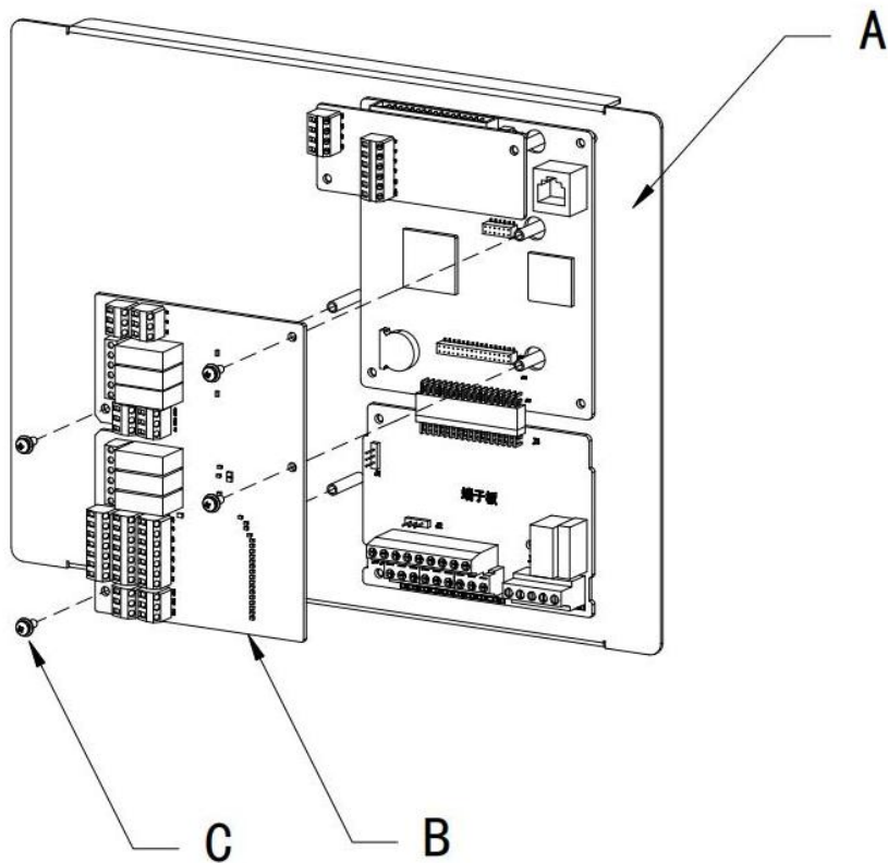
A: 钣金支撑件 B: 工艺卡 C: 螺钉
