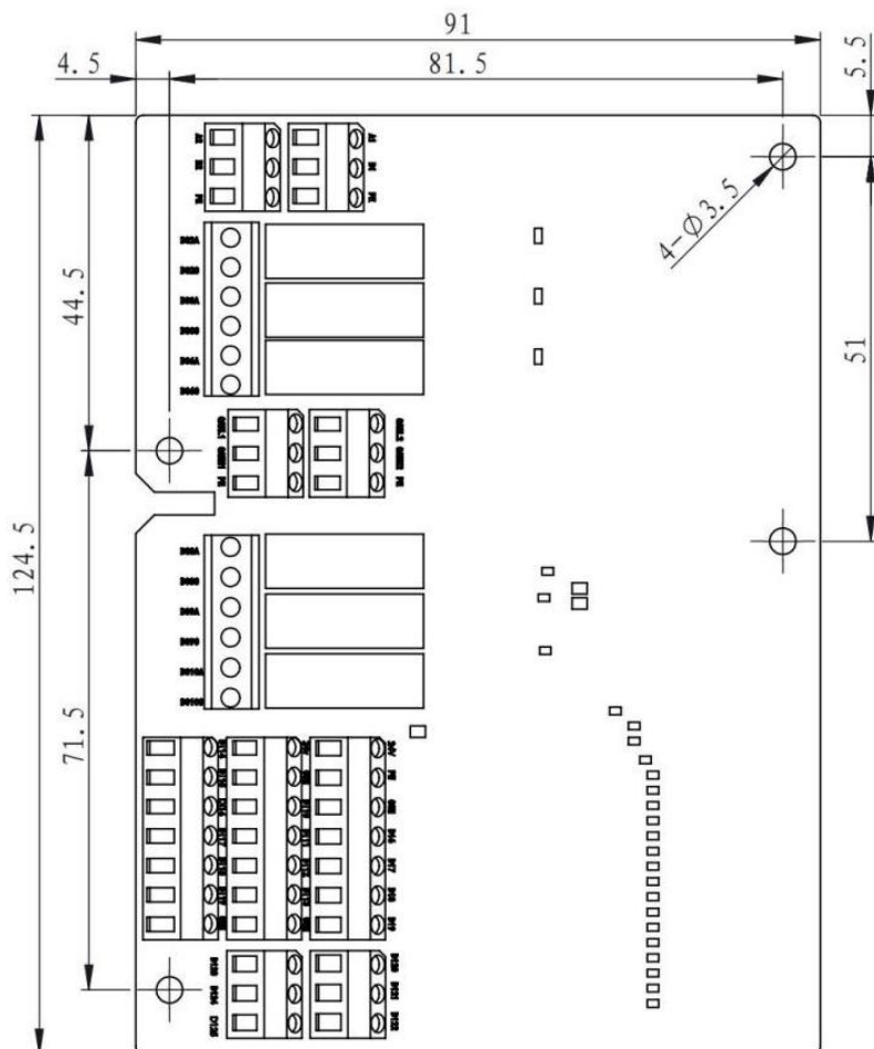
GDHF-AGYZ1 工艺卡尺寸 (单位 mm)
